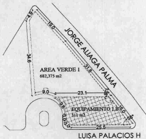
SITUACION PROPUESTA (AREA VERDE 1 Y EQUIPAMIENTO 1B)
