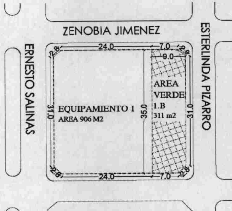
SITUACION PROPUESTA (EQUIPAMIENTO 1 Y AREA VERDE 1B) ESC. 1/500
